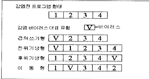
그림 2. 바이러스 감염 전·후 형태변화 Fig 2. Change of file structure after the infection of a virus.
