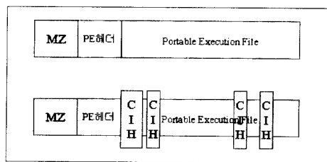
그림 9. CIH 감염 파일의 CIH 분할정보(상단-감염전, 하단-감염후) Fig 9. Partial CIH informations in CIH infected file (top-before infection, down-infected)
