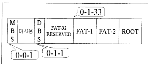
그림 11. 윈도95의 파일 시스템의 정보 영역 Fig 11. Information area of Windows '95 file system.
