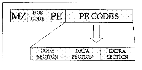
그림 6. PE의 구조 Fig 6. The structure of PE-file
