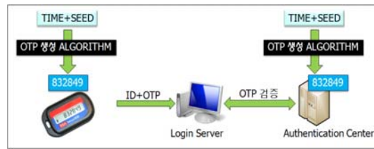
[그림 1] OTP 인증 과정
